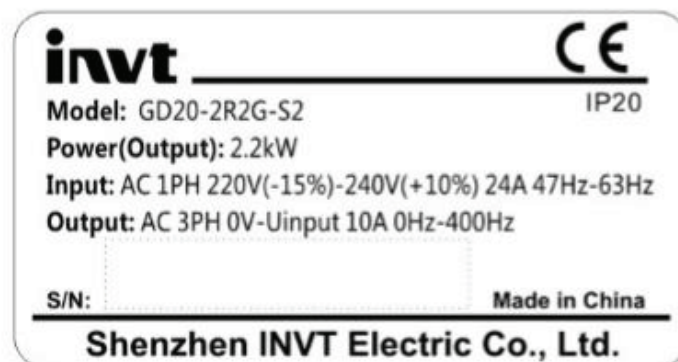
Hình 2-1 Bảng tên
