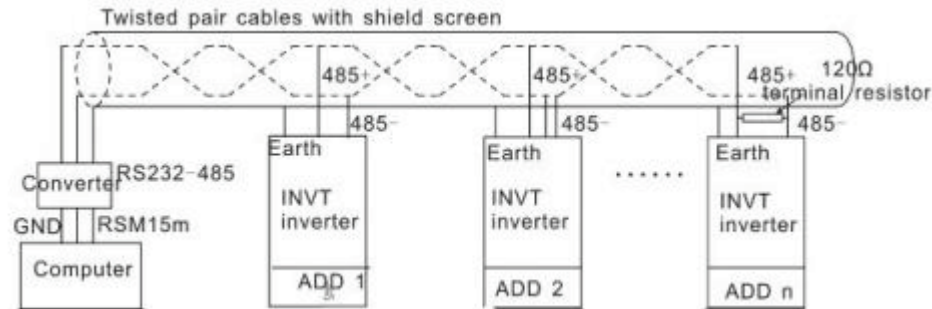
Hình 2: Truyền nối tiếp
