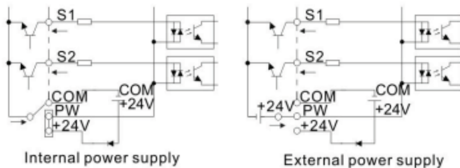
Hình 3-12 Kiểu NPN
