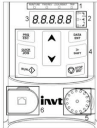
Hình 4-1: Bàn phím
