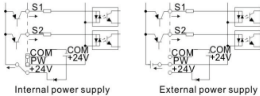
Hình 3-13 Kiểu PNP
