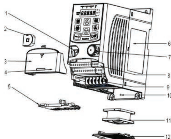
Hình 2-3 Cấu trúc sản phẩm (3PH 380V, \leq 2.2kW )
