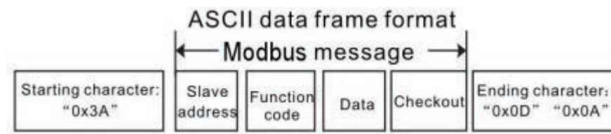
Định dạng khung truyền ASCII
