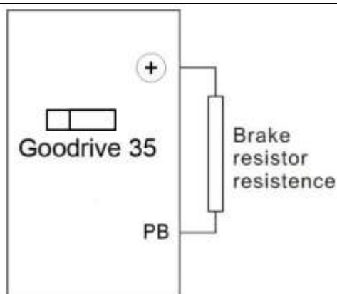
Lắp đặt bộ hãm động năng
