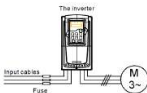
Hình 4-25 Cấu hình cầu chì
