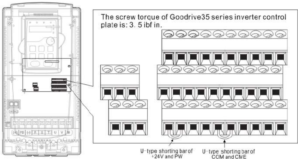
Hình 4-22 Cầu nối U
