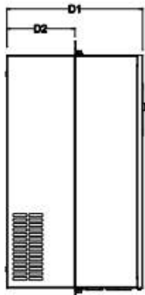
Lắp đặt trên tường biến tần 380V 37 – 110 kW
