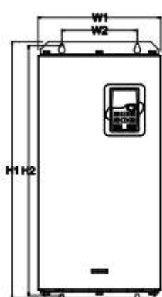
Lắp đặt trên tường biến tần 380V 37 – 110 kW
