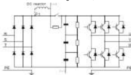
Hình 3-3 Sơ đồ mạch chính đơn giản hóa (biến tần 660 V)
