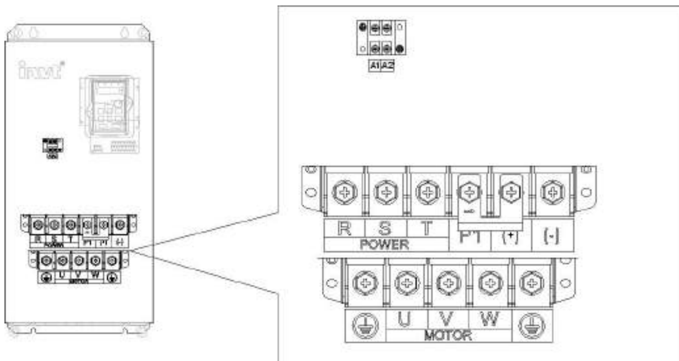
Hình 4-14 : sơ đồ ngõ Terminal của hệ thống biến tần 380 có công suất 75~110Kw
