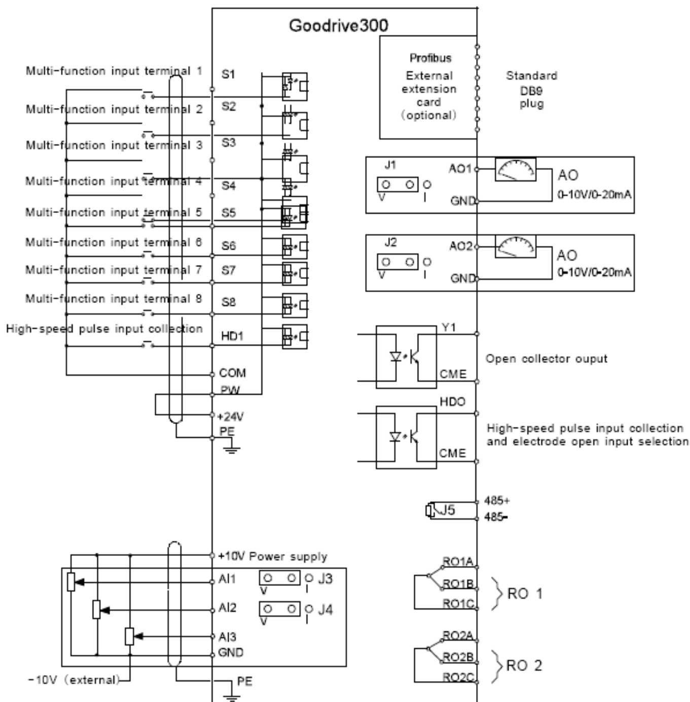
Hình 4.20 Sơ đồ đấu dây mạch điều khiển
