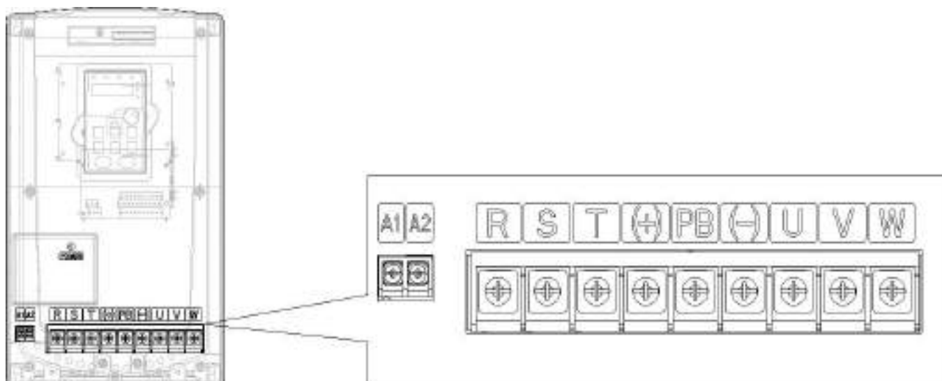
Hình 4-12 : sơ đồ ngõ Terminal của hệ thống biến tần 380 có công suất 22~30Kw
