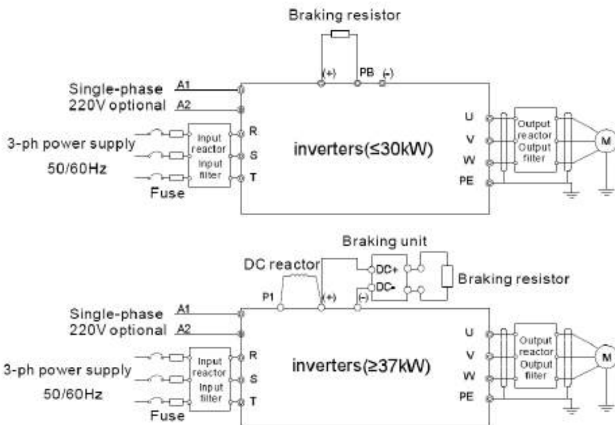
Hình 4.7 Sơ đồ kết nối mạch chính cho biến tần 380V
