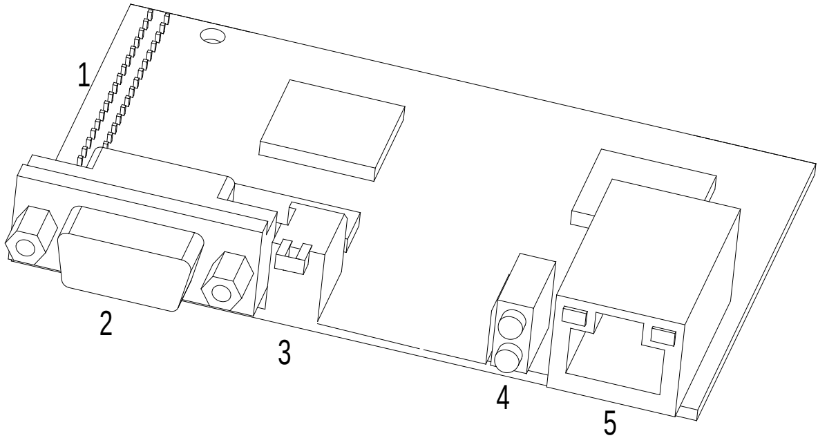
Sơ đồ cấu trúc bên ngoài của EC-TX-103
