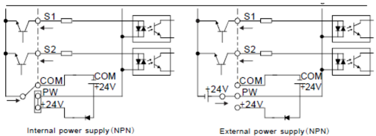
Hình 4.23 Chế độ NPN
