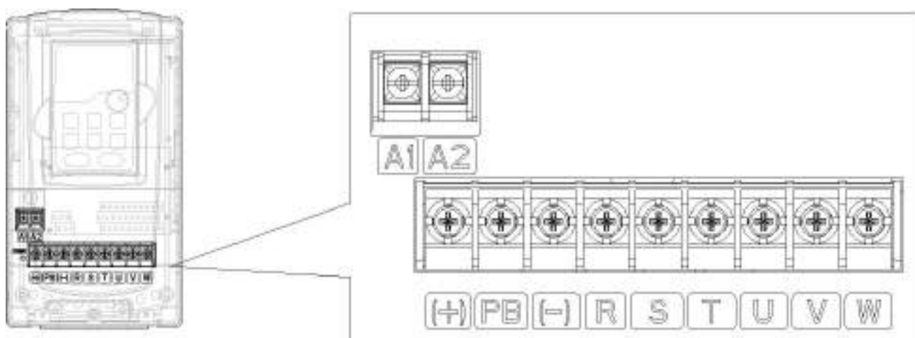
Hình 4-10 : sơ đồ ngõ Terminal của hệ thống biến tần 380 có công suất 7.5~11Kw
