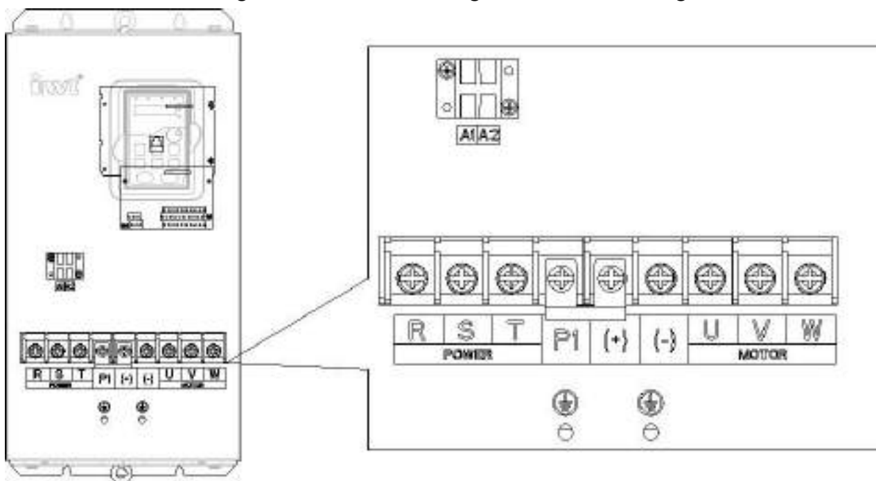
Hình 4-13 : sơ đồ ngõ Terminal của hệ thống biến tần 380 có công suất 37~55Kw
