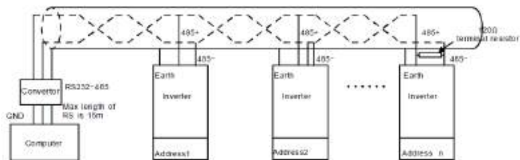
Hình 2 : Truyền nối tiếp
