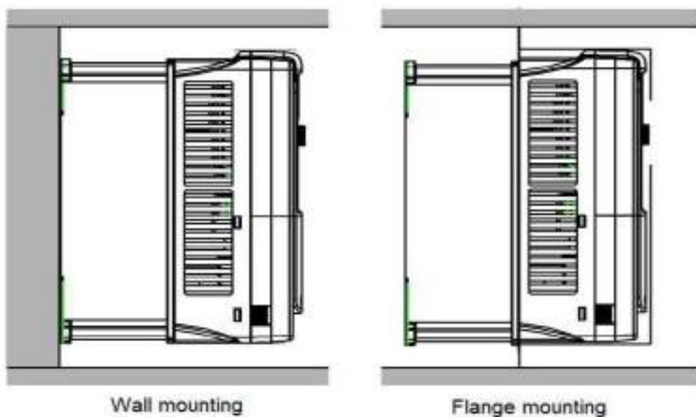
4-2 : Vị trí lắp đặt
