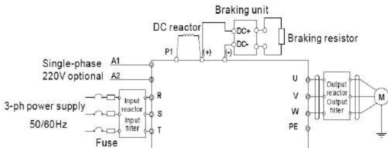
Hình 4.10 Sơ đồ kết nối mạch chính cho biến tần 660V
