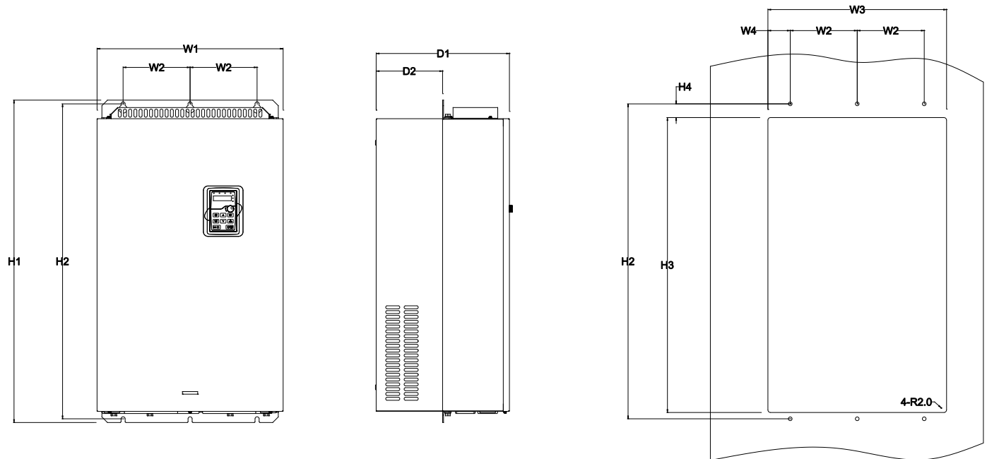
Lắp đặt âm tường cho loại 660V 160~220 Kw
