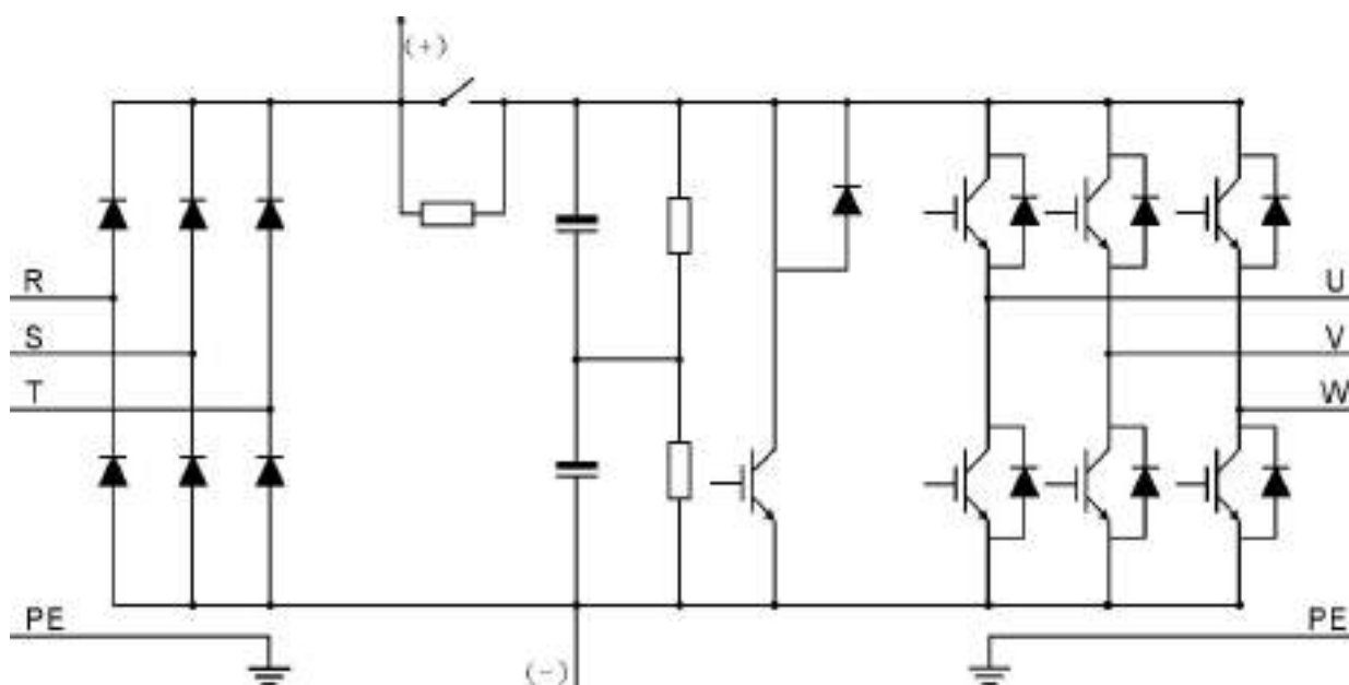
Hình 3-1 : sơ đồ mạch chính của dòng biến tần \geq 37\text{Kw}
