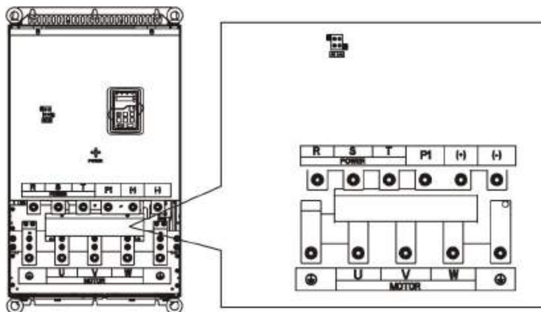
Hình 4-15 : sơ đồ ngõ Terminal của hệ thống biến tần 380 có công suất 132~200Kw
