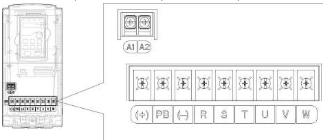
Hình 4-11 : sơ đồ ngõ Terminal của hệ thống biến tần 380 có công suất 15~18Kw
