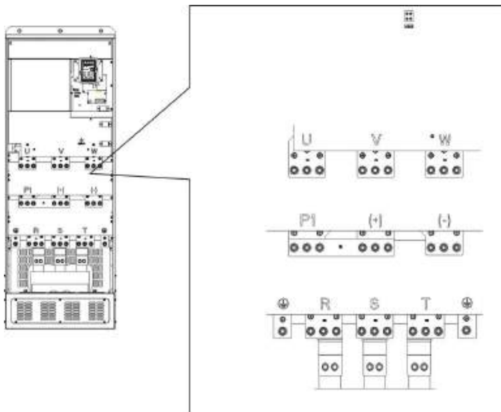
Hình 4-17 : sơ đồ ngõ Terminal của hệ thống biến tần 380 có công suất 350~500Kw
