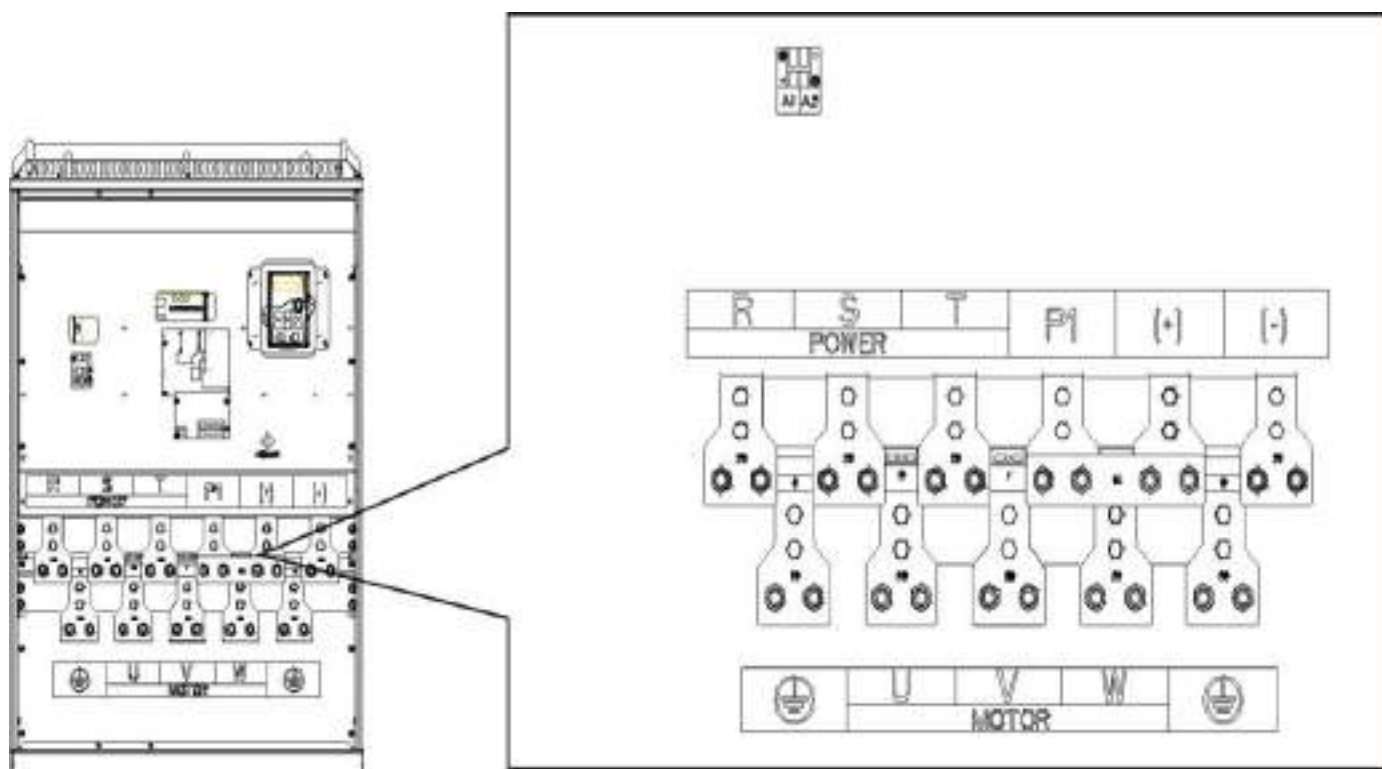
Hình 4-16 : sơ đồ ngõ Terminal của hệ thống biến tần 380 có công suất 220~315Kw
