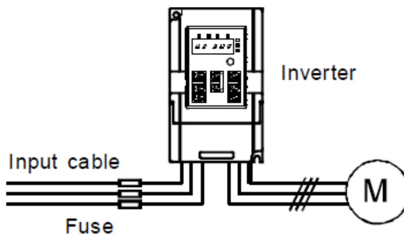
Hình 4-25 : Cầu chì bảo vệ
