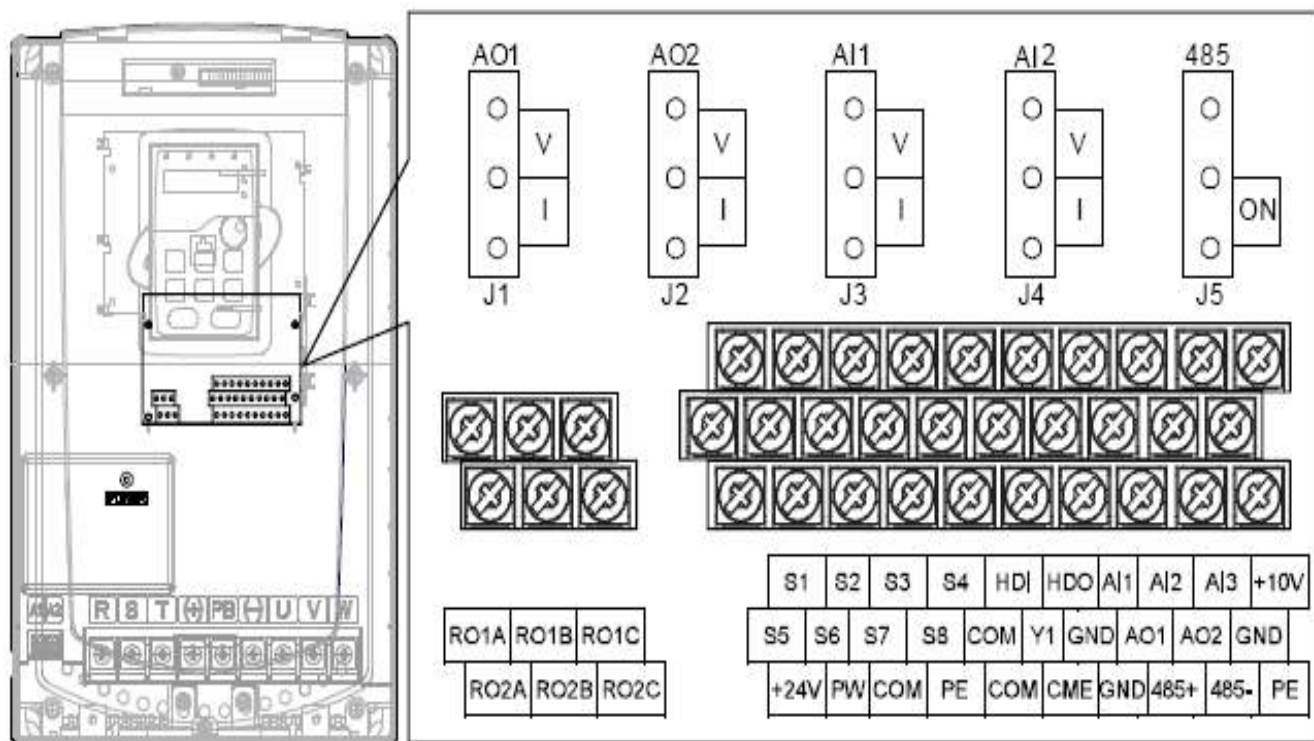
Hình 4.2 Terminal mạch điều khiển
