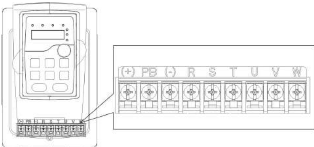
Hình 4-8 : sơ đồ ngõ Terminal của hệ thống biến tần 380 có công suất 1.5~2.2Kw
