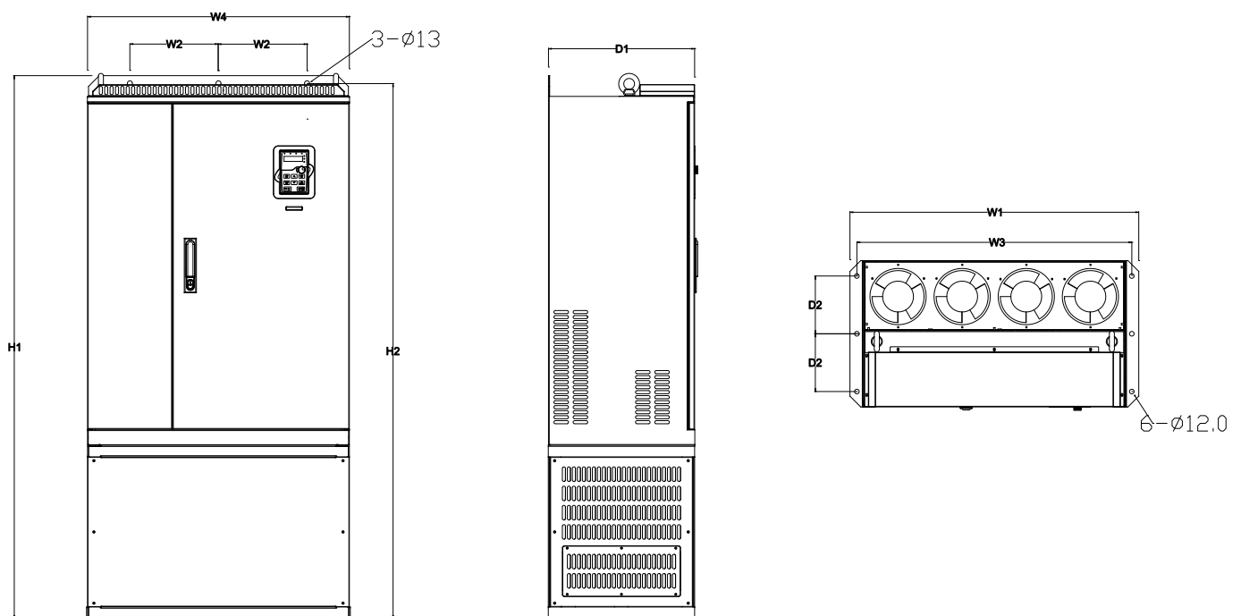
Lắp đặt trên sàn cho loại 660V 250~350 Kw
