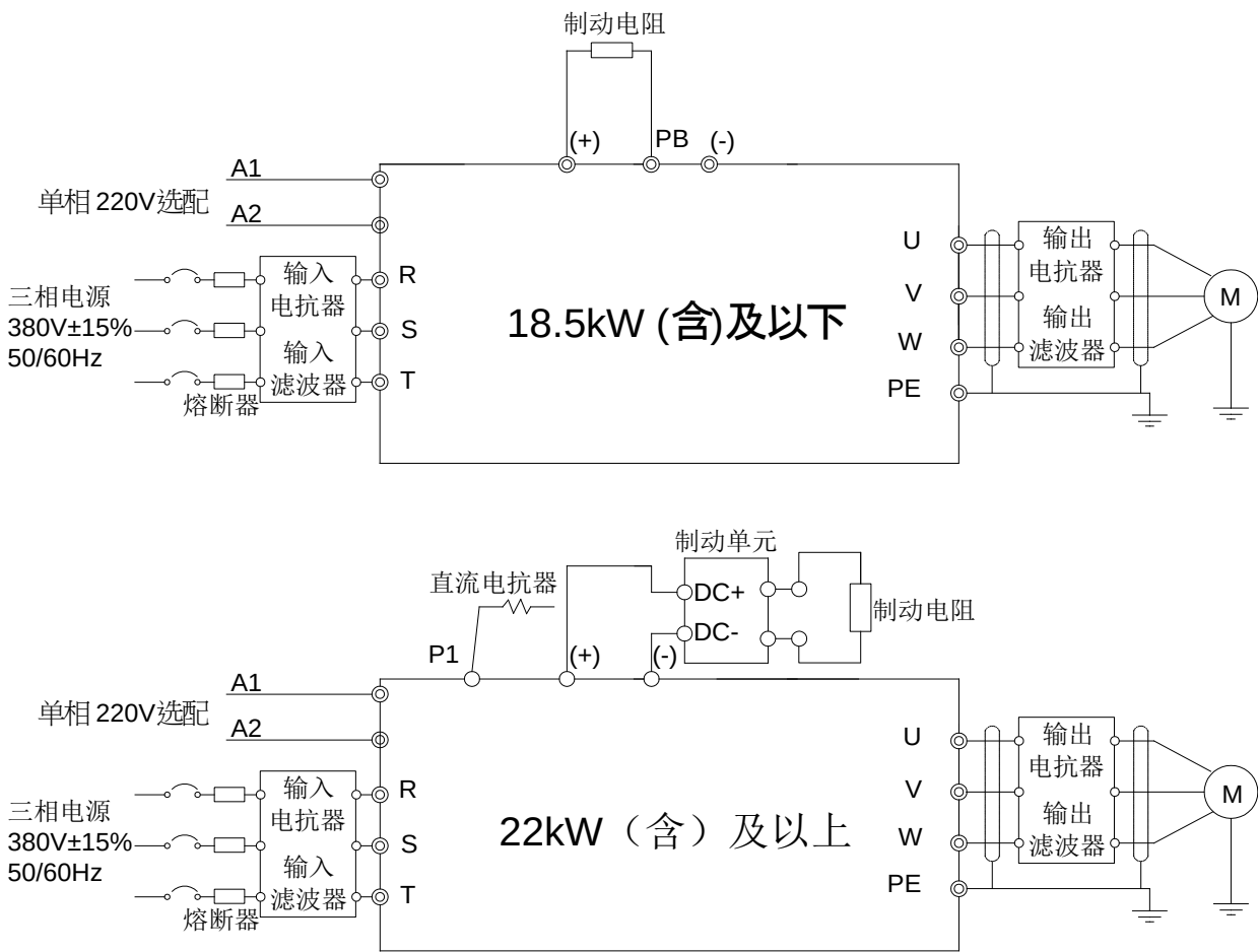
Hình 4.9 Sơ đồ kết nối mạch chính cho biến tần 550V
