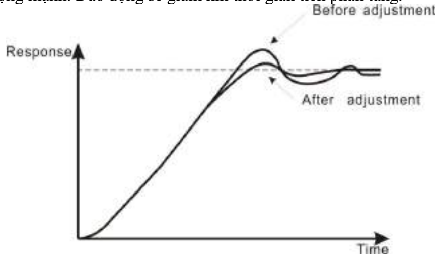
Hình 6.26 Giảm dao động chu kỳ dài.
