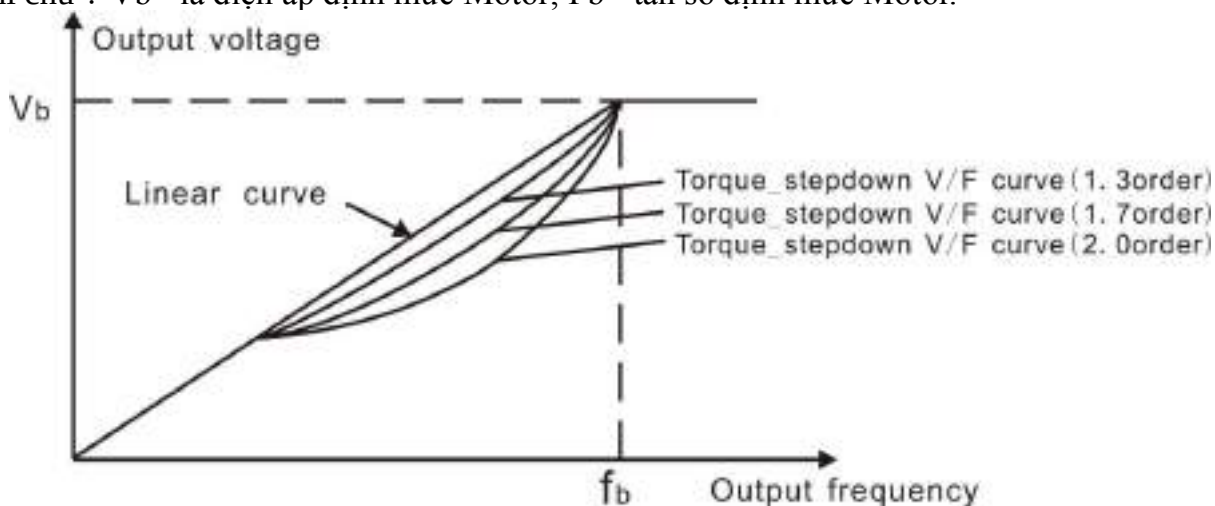
Hình 6.8 Biểu đồ các đường đặc tuyến V/F.
