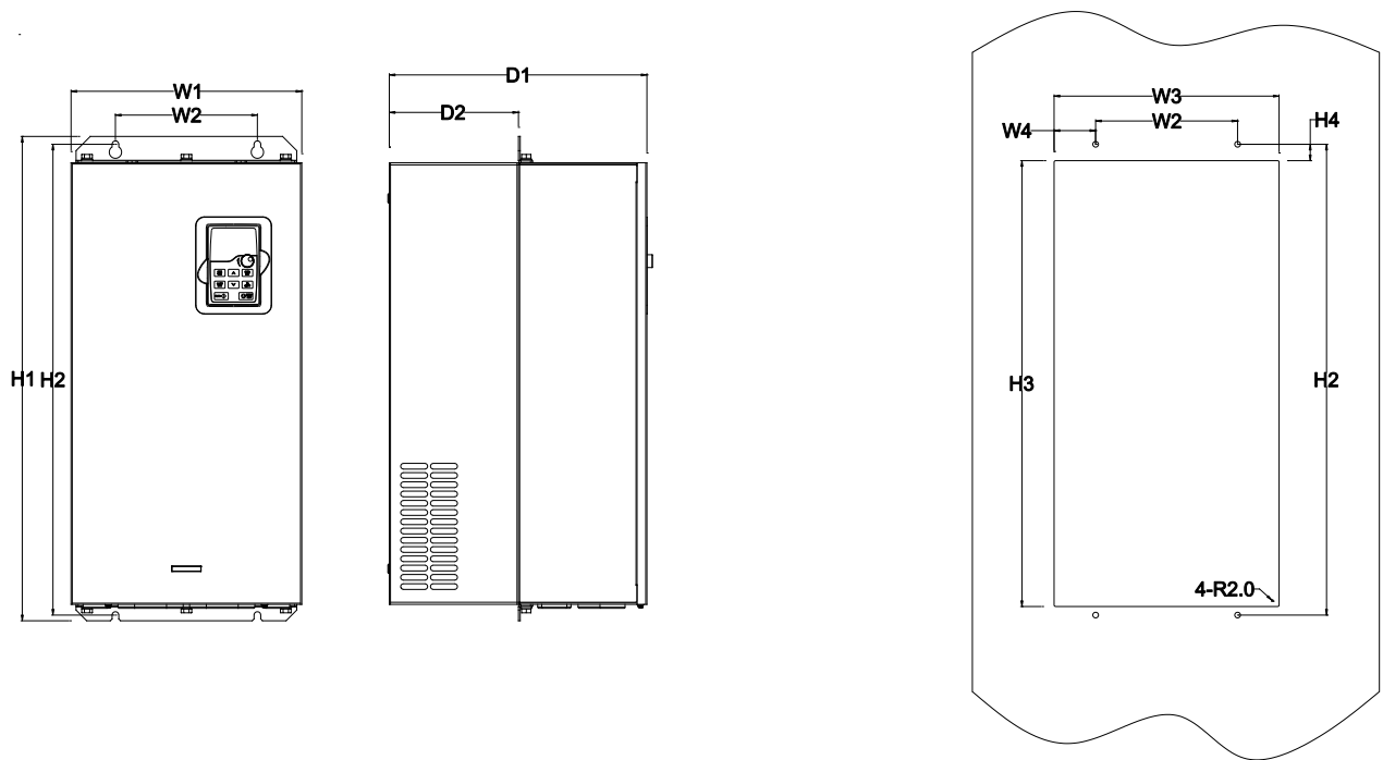
Lắp đặt âm tường cho loại 660V 22~132Kw
