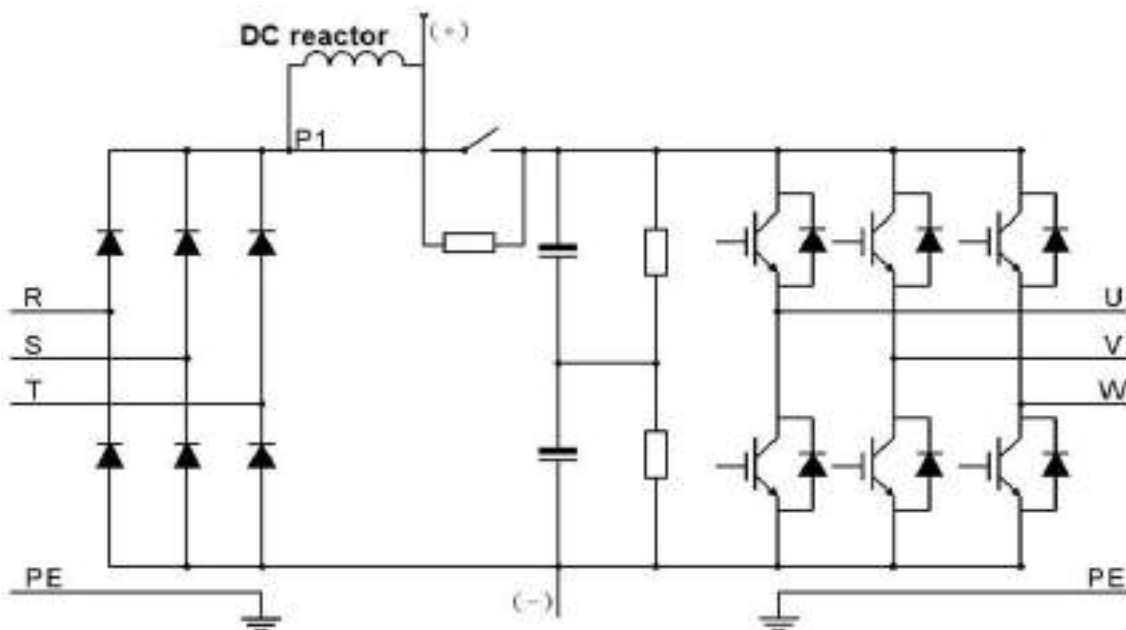
Hình 3-1 : sơ đồ mạch chính của dòng biến tần ≤30Kw
